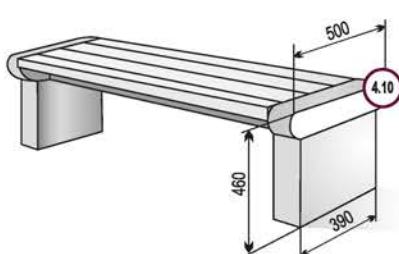
4.10 СКАМЕЙКА
