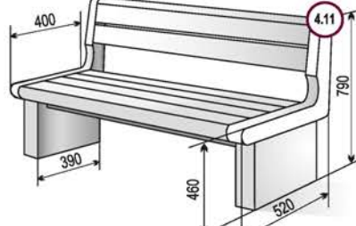
4.11 СКАМЕЙКА
